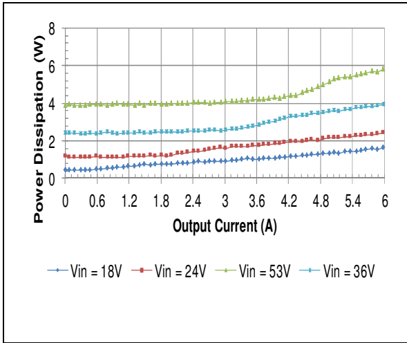
V_o = 15V
