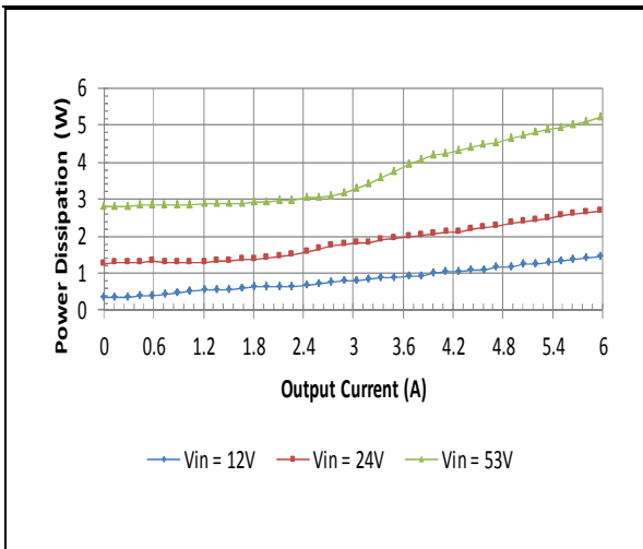
V_o = 9.6V
