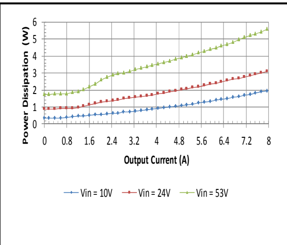
V_o = 5V
